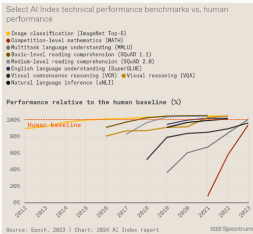
Figura 7: Rendimiento IA vs Humano
