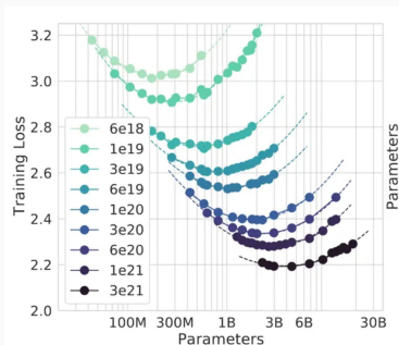
Figura 14: Límites
