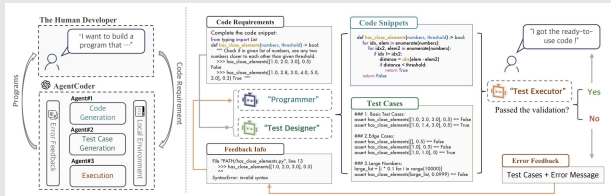
Figura 16: Agentes
