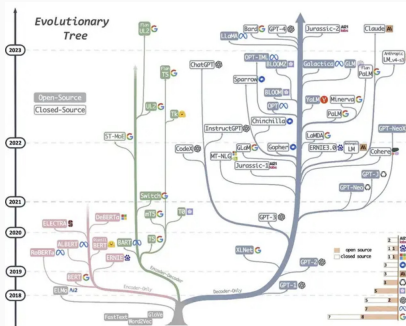
Figura 3: Arbol
