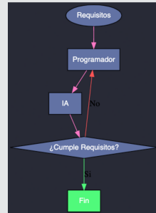
Figura 20: Modelo desarrollo
