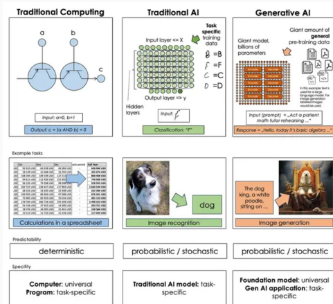
Figura 2: Evolución IAS
