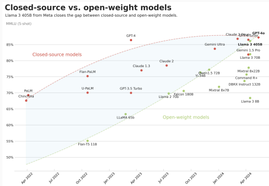
Figura 13: Resultados test open vs close
