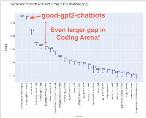
Figura 12: Resultados en Codificación
